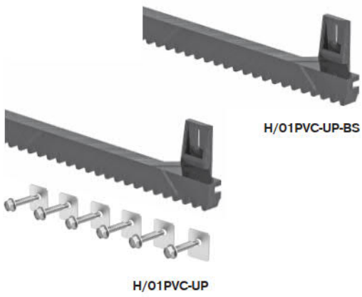
H/01PVC-UP
