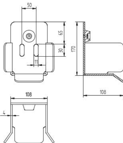
H/16-46x130 H8/16-46x130
